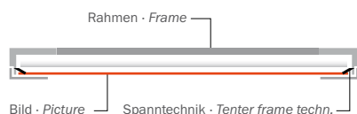
Leuchtkasten Spanntechnik mit Klapprahmen Tenter lightbox with hinged alternate frame
