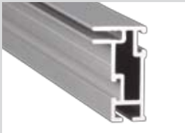
Slim-Frame „25“ Profil rahmenlose Optik Bautiefe: 25 mm Ausführung: 1-seitig
